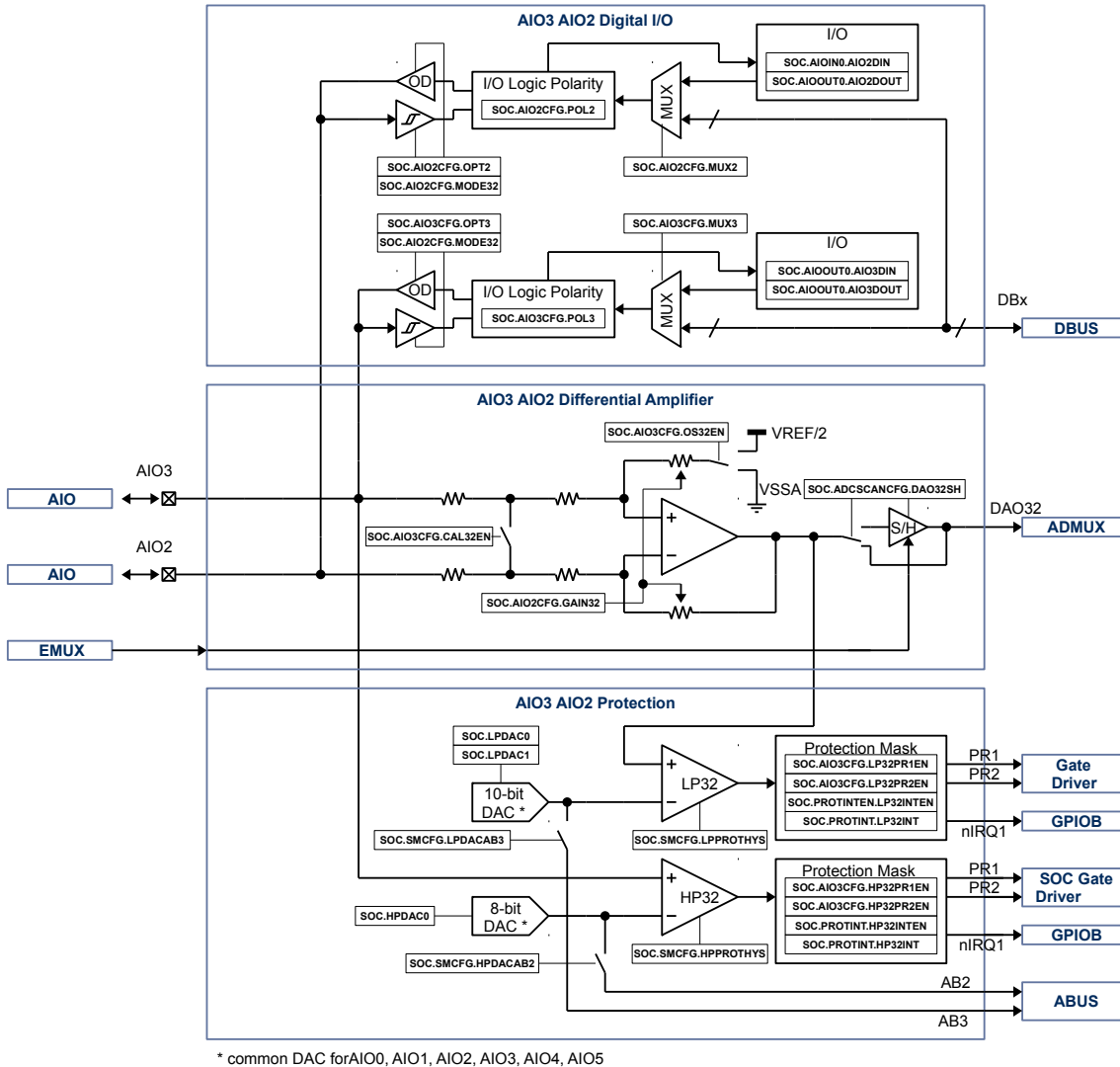
Figure 22-3. AIO3, AIO2
