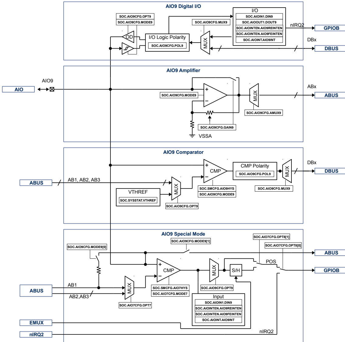
Figure 22-8. AIO9
